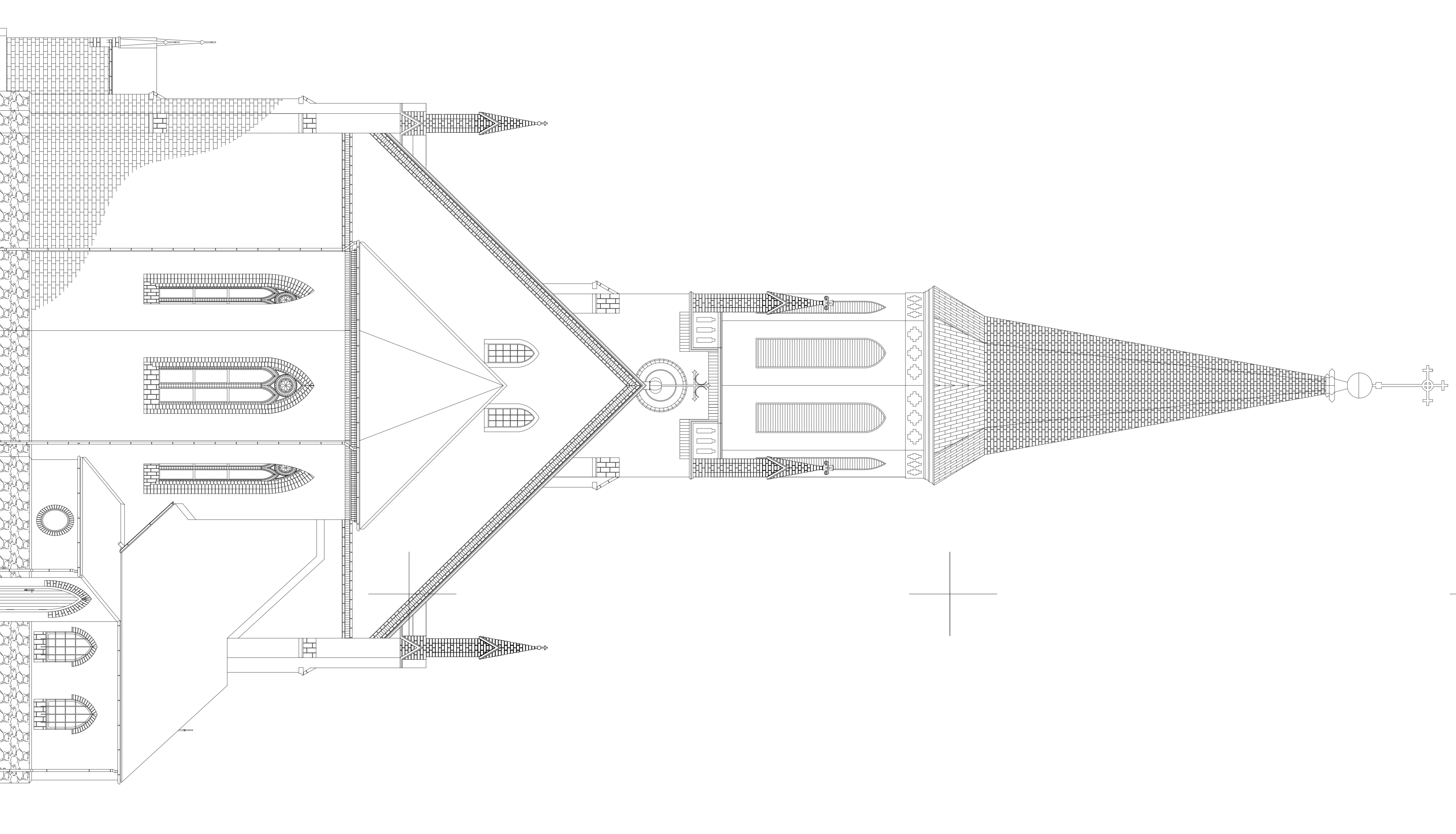
ELEWACJA C-D
