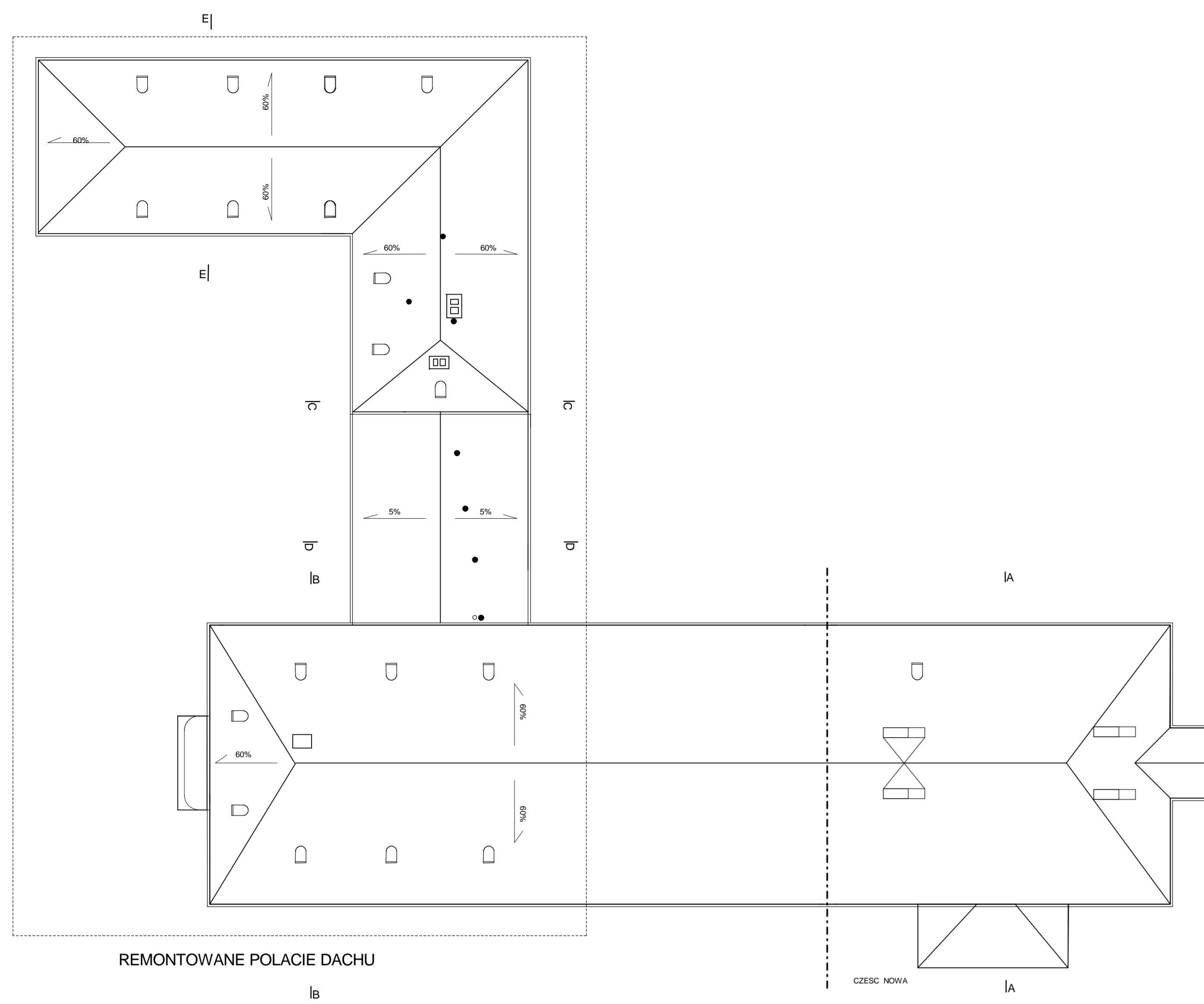
RZUT DACHU 1 : 200 projekt
