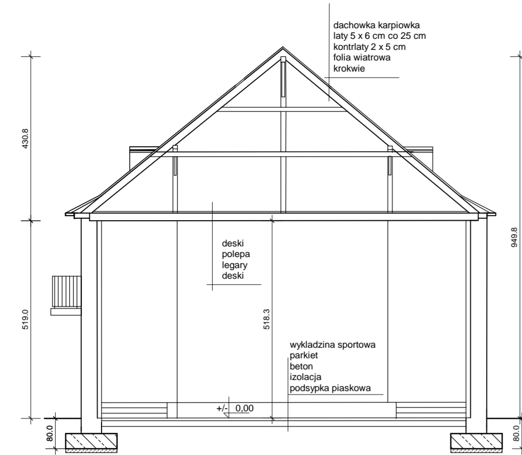
PRZEKRÓJ E - E 1 : 100
