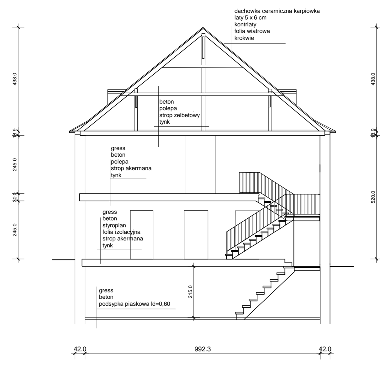
PRZEKRÓJ D - D 1 : 100
