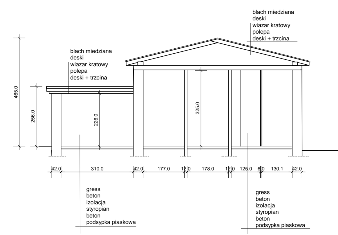
PRZEKRÓJ C - C 1 : 100
