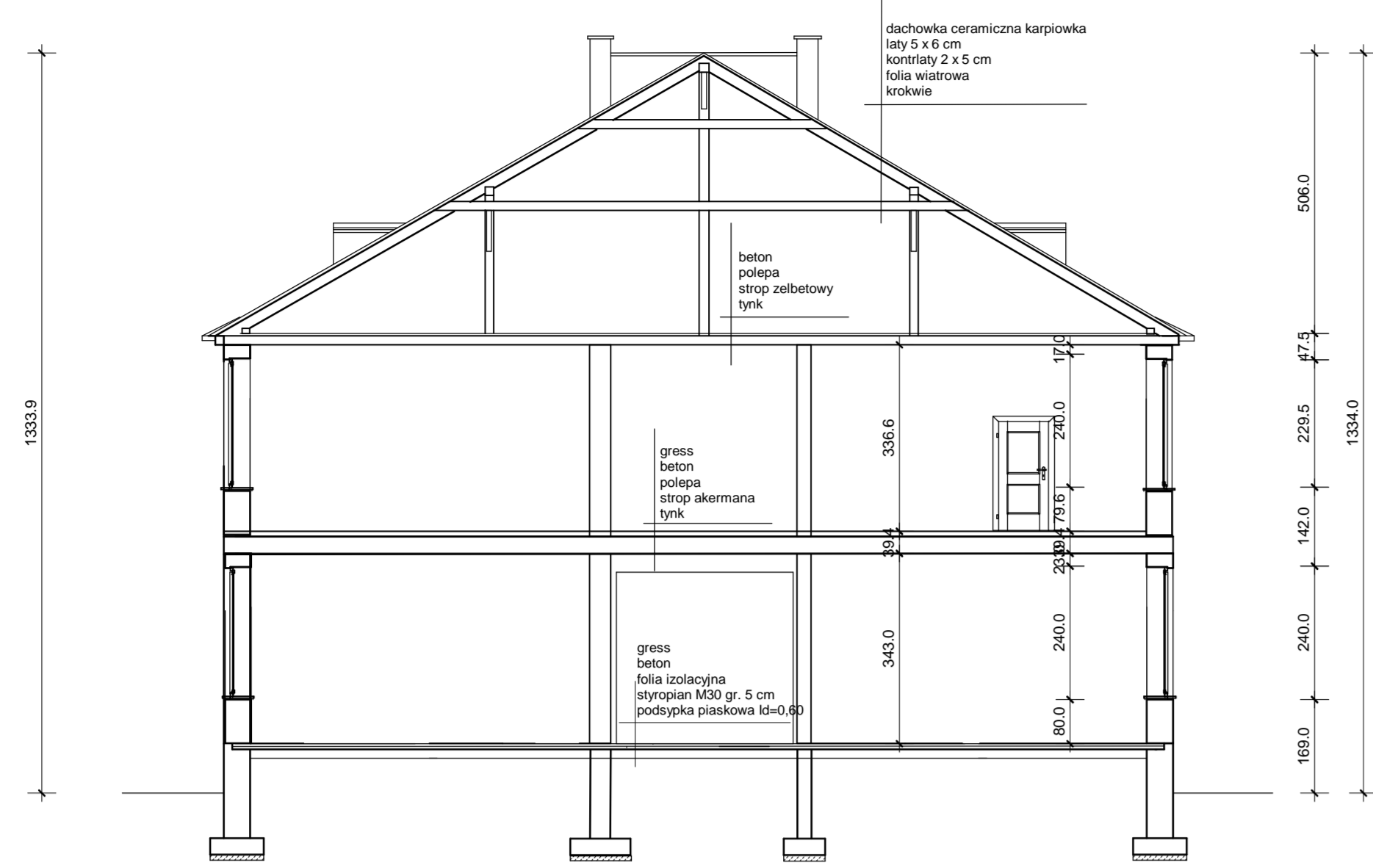
PRZEKRÓJ B - B CZ. A 1 : 100
