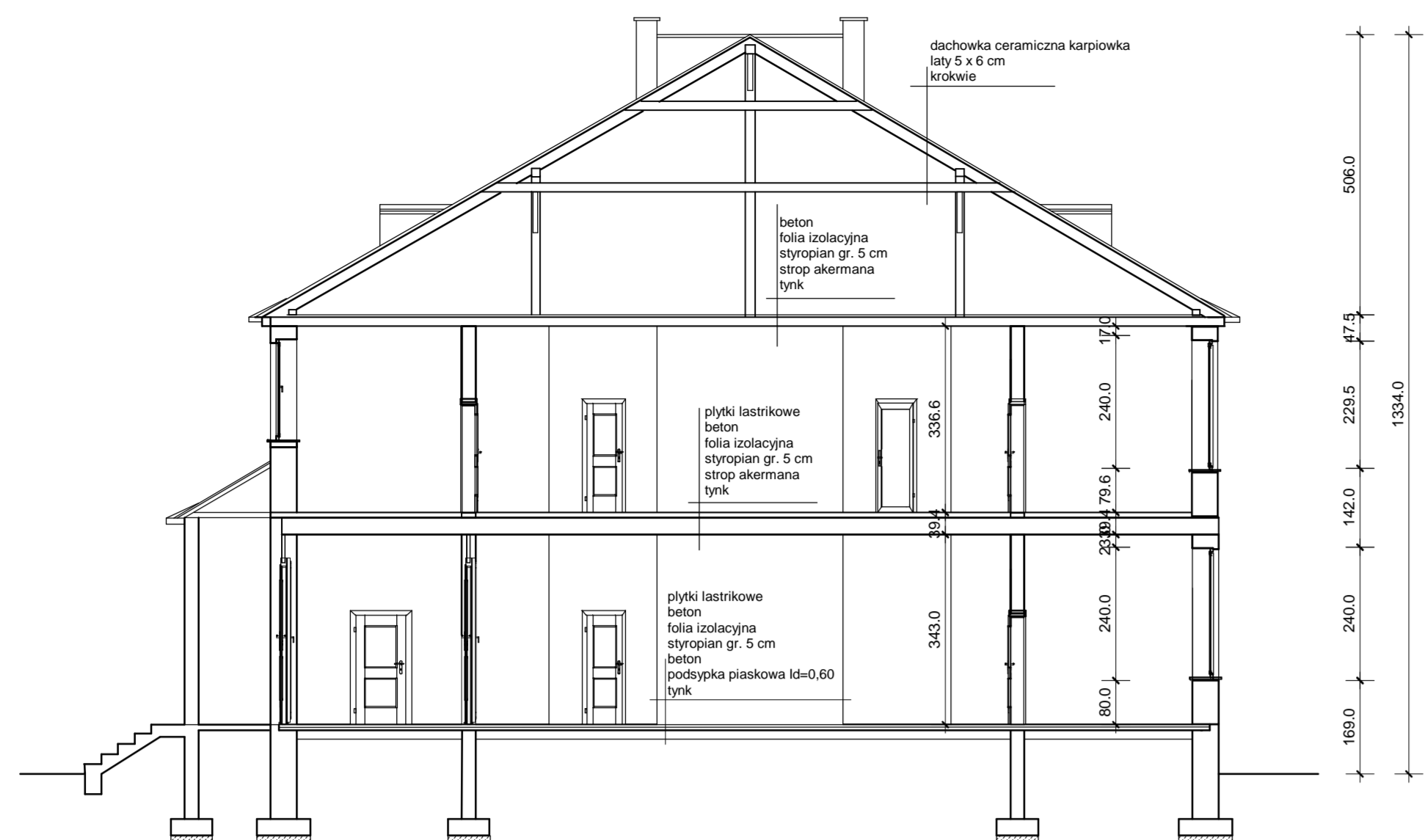
PRZEKRÓJ A - A CZ. A 1:100
